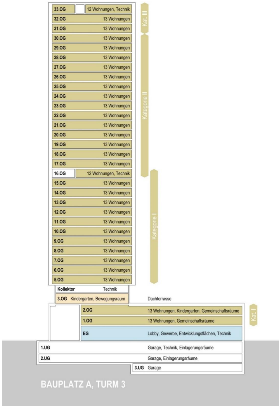
Gebäudeschnitt
